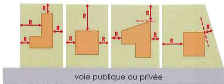
R = recul aux limites séparatives
